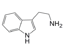
Tryptamine
