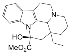
Vincamine
