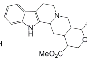
Ajmalicine
